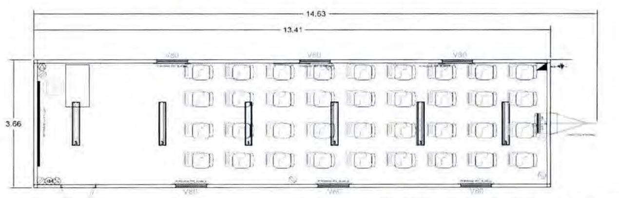
Aula en lámina de 12 x 48 (de 3.64 mts de ancho x 13.41 mts de largo + 1.22 mts de jalón)
